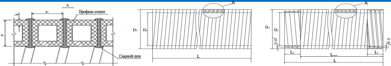
Спиральнолитые трубы «ТЕХСТРОЙ СВТ» Тип 1 (а) и Тип 2 (с внутренней и с наружной резьбой) (б)
