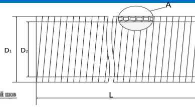
Спиральновитые трубы «ТЕХСТРОЙ СВТ» Тип 1 (а) и Тип 2 (с внутренней и с наружной резьбой) (б)
