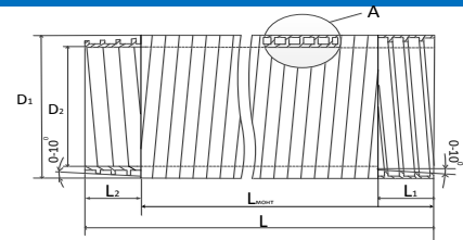
Спиральновитые трубы «ТЕХСТРОЙ СВТ» Тип 1 (а) и Тип 2 (с внутренней и с наружной резьбой) (б)
